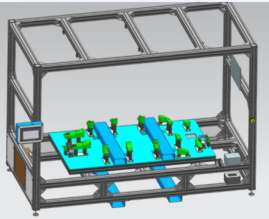
影像检测夹具
