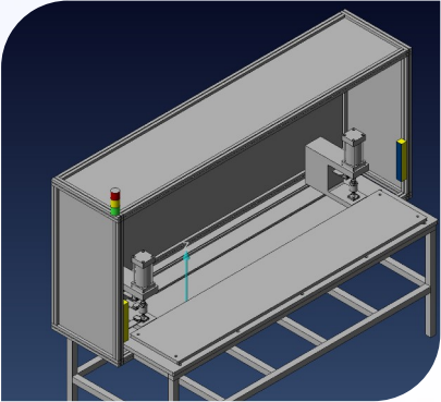
卡扣装配夹具
